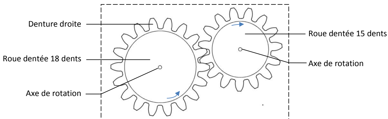
Croquis d'un engrenage à denture droite
